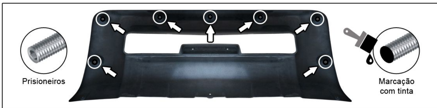
C) Inserir os 7 prisioneiros nos insertos da peça conforme locais indicados. Em seguida, fazer uma marcação com tinta na ponta dos prisioneiros (essa marcação serve p/ verificar os locais de furação do para-choque conforme etapa seguinte).
